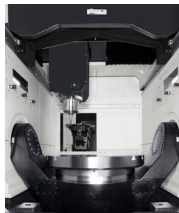
Takumi U 800: Schwenkbrücke von Kessler mit drei Torque-Antrieben
